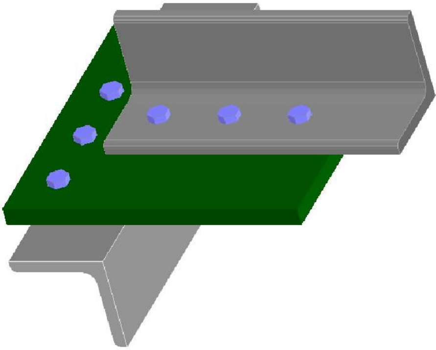
Collegamento piastra di rinforzo (reticolare singola)
