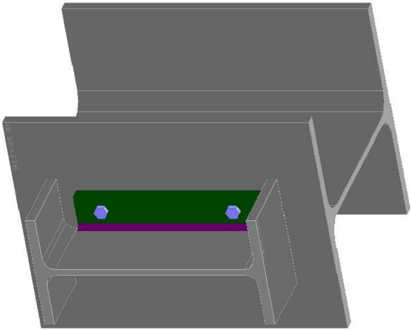
Collegamento colonna-trave (flangiato)
